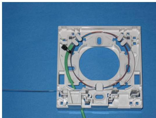
Směr zatočení optického kabelu
