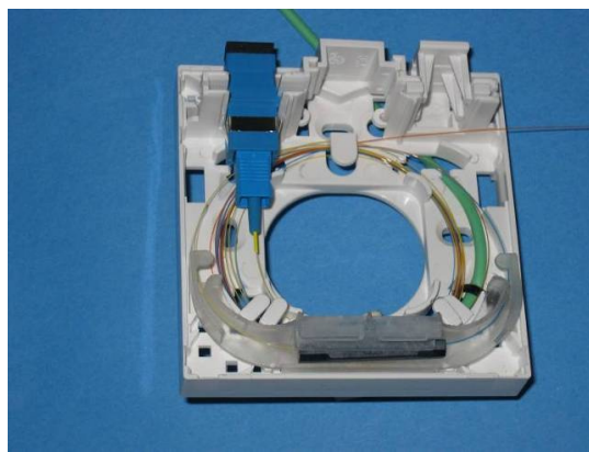
Umístění prvního optického pigtailu a spoje
