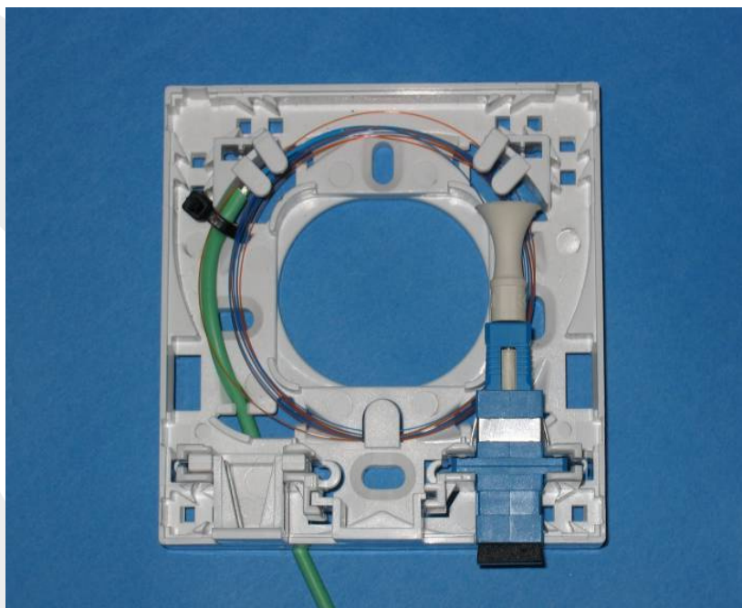
Přímé ukončení SC konektorem
