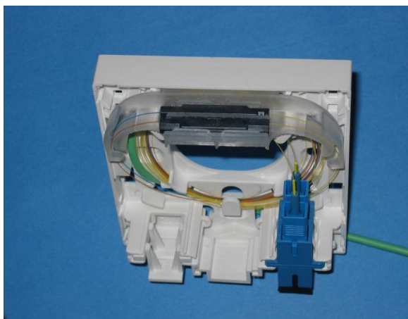
Umístění druhého optického pigtailu a spoje
